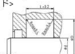
<ロータリー>
